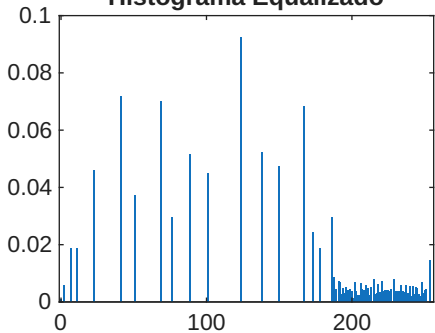
Histograma Equalizado
